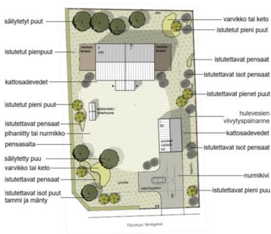
Kuva 24. Ideakuva pihasuunnitelmasta (tontin pinta-ala 2300 m²)
